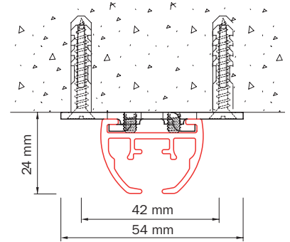
plafondmontage met plafondsteun 6055-1000
