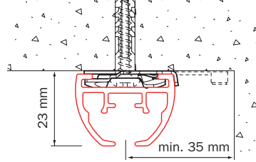
plafondmontage met spanner 6050
